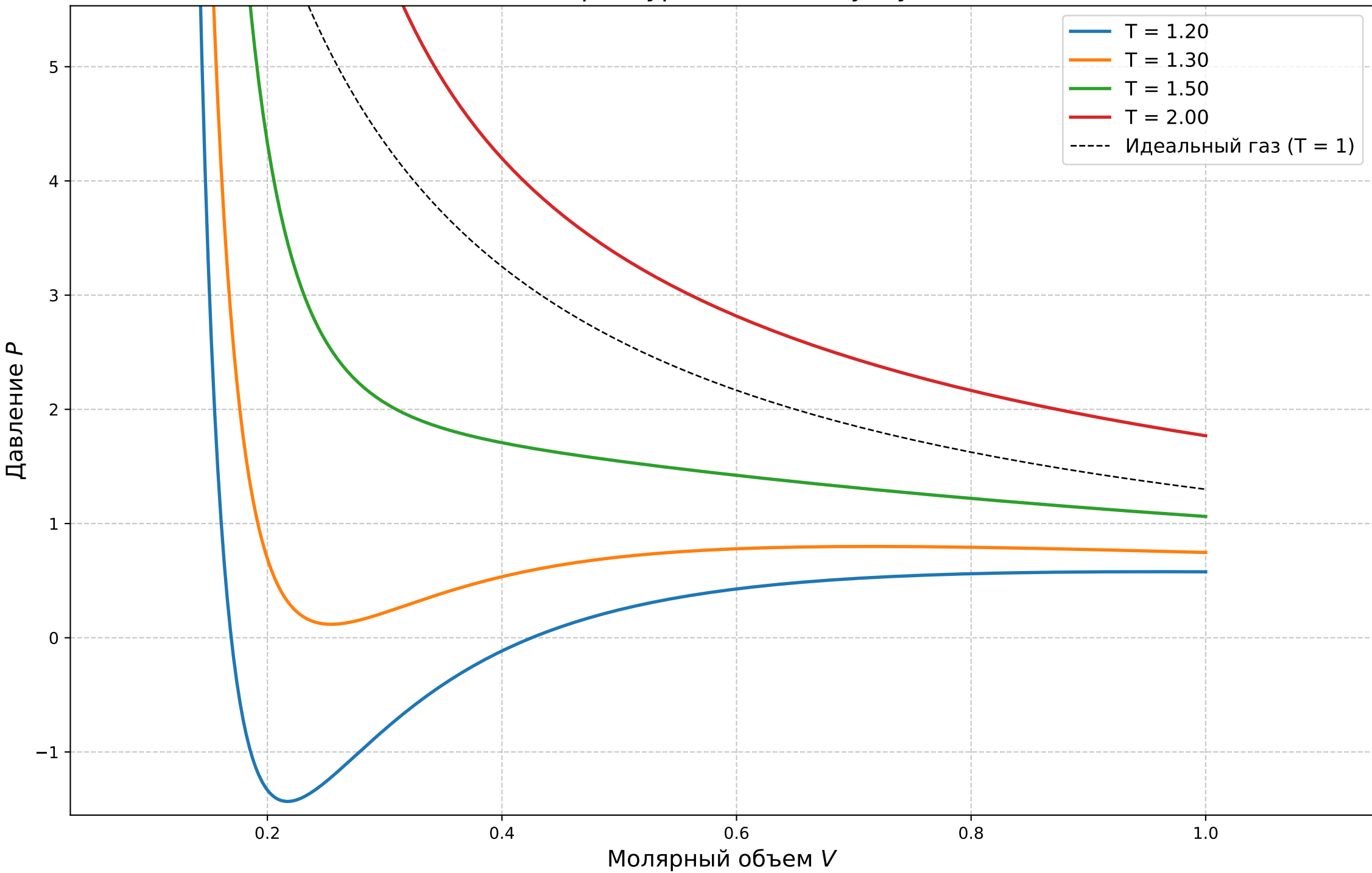
Изотермы уравнения Клаузиуса
